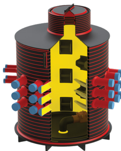
Колодец с защитным огнестойким внутренним слоем**
